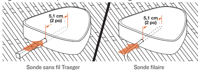
Sonde sans fil Traeger
